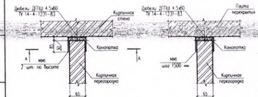
РАЗРЕЗ А-А
